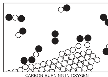
图 1.8: 碳在氧气中的燃烧
